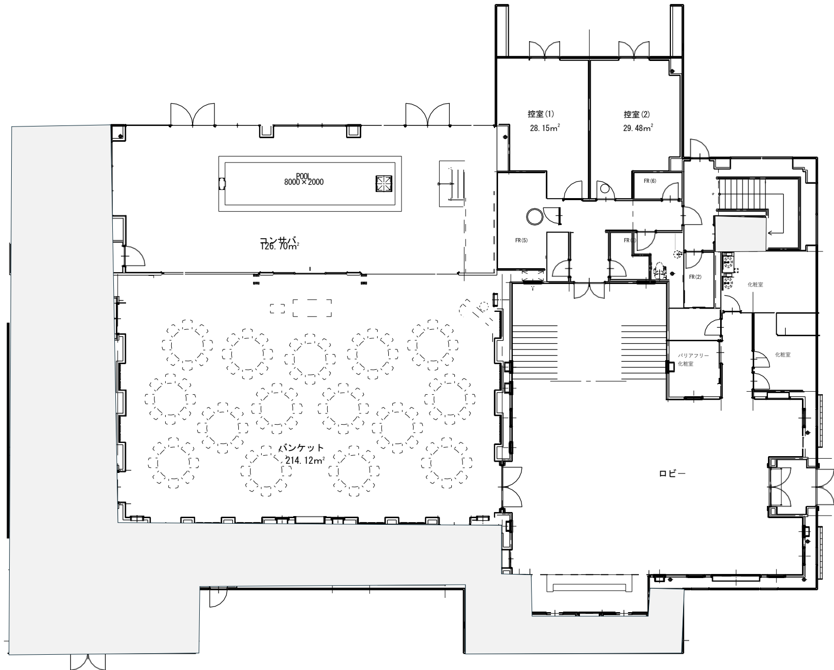
NEEDS札幌 平面図 (1F)
