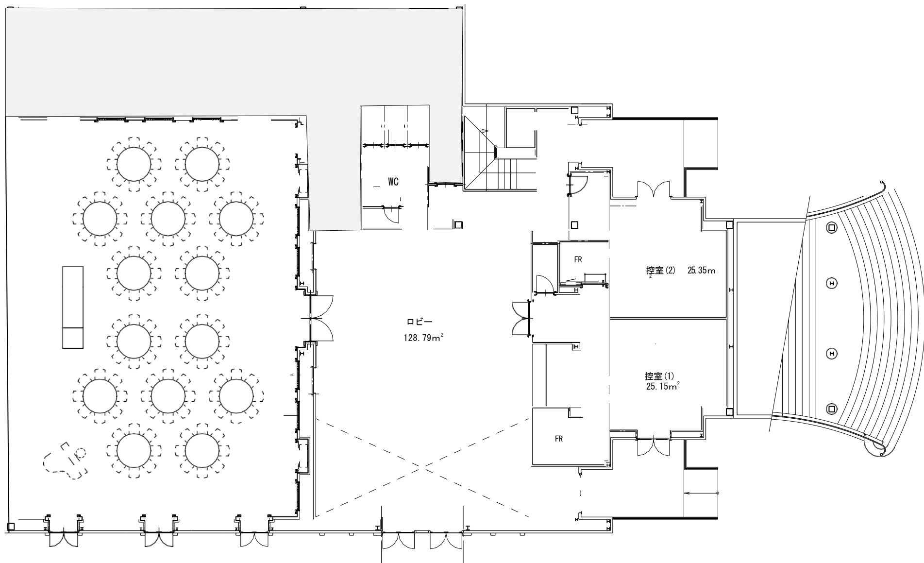
ベイスайд迎賓館和歌山 ホワイトハウス 1F
